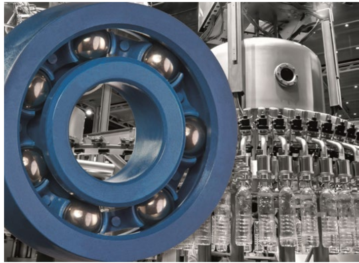
图片注解 1615-01： 来自易格斯的 xiros 工程塑料轴承免润滑、免维护。 xiros M180 还可侦测，抗化学介质。
